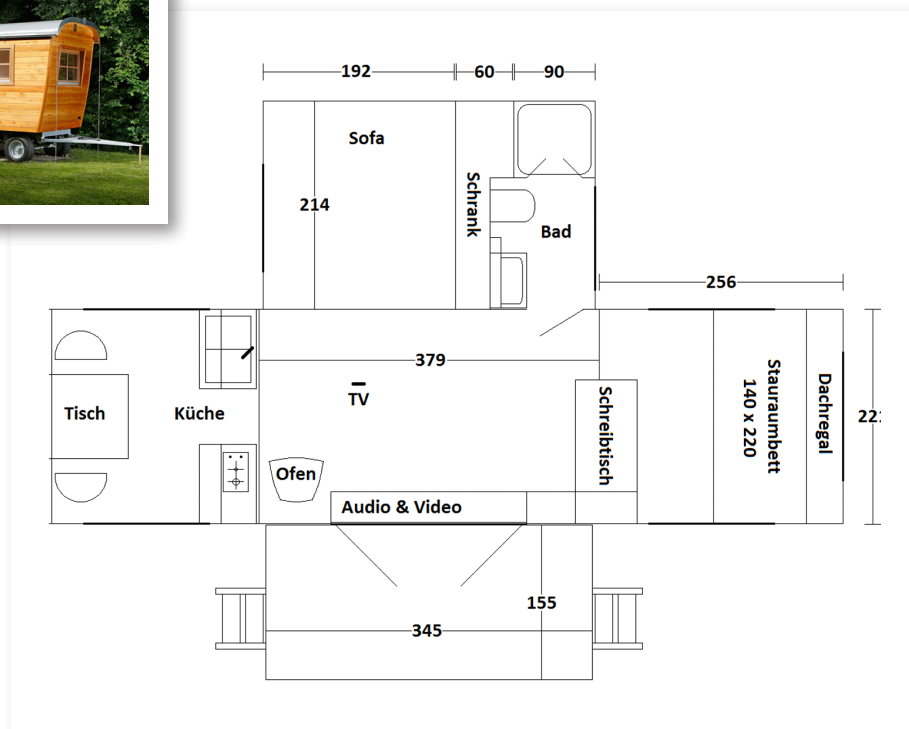
Grundriss Wohlwagen L. Innenmaße in cm.
