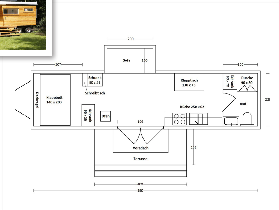
Grundriss Wohlwagen M. Innenmaße in cm.
