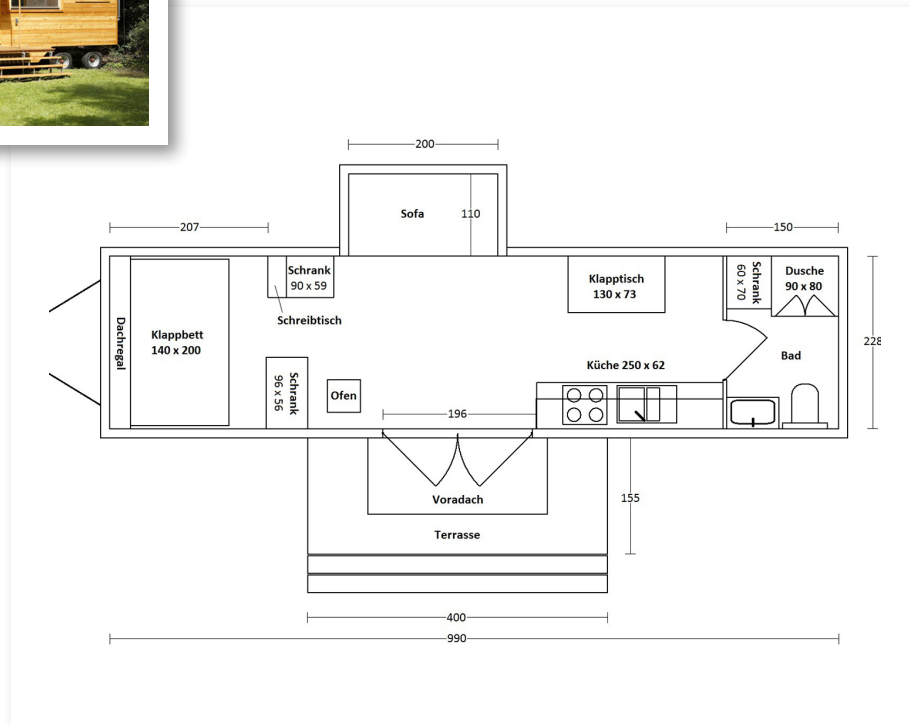
Grundriss Wohlwagen M. Innenmaße in cm.
