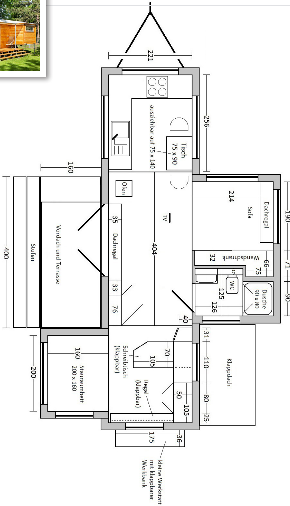
Grundriss Wohlwagen L2. Innenmaße in cm.
