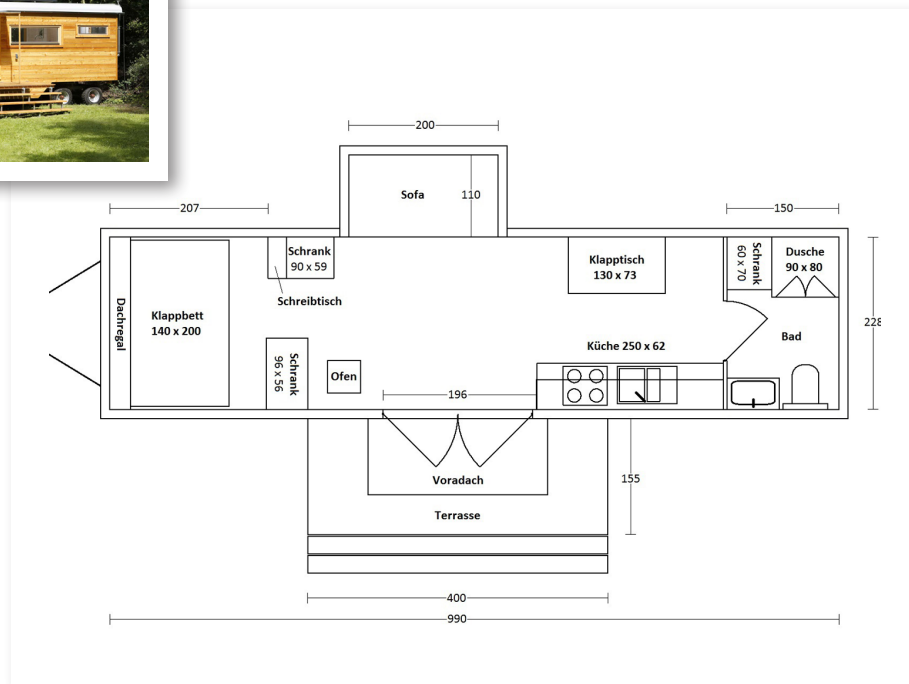
Grundriss Wohlwagen M1. Innenmaße in cm.
