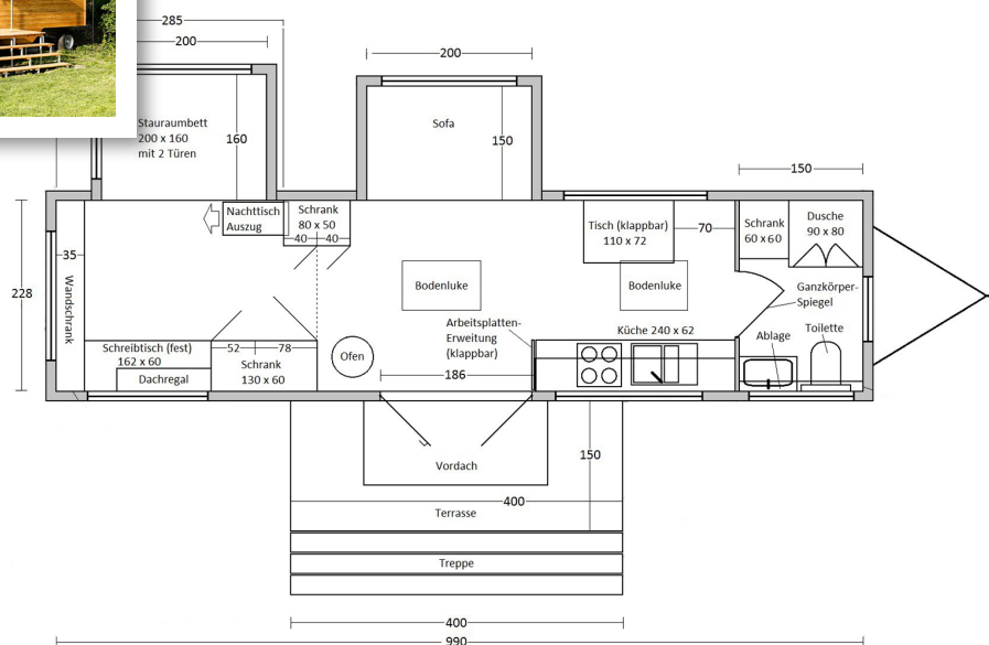
Grundriss Wohlwagen M2. Innenmaße in cm.
