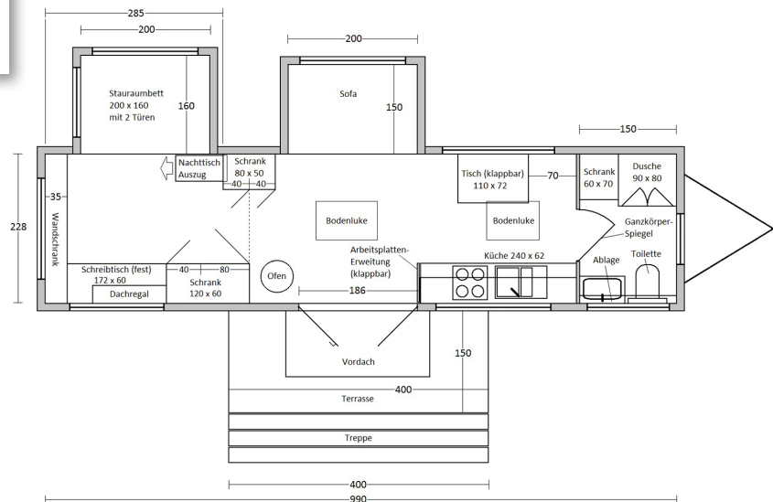
Grundriss Wohlwagen M2. Innenmaße in cm.
