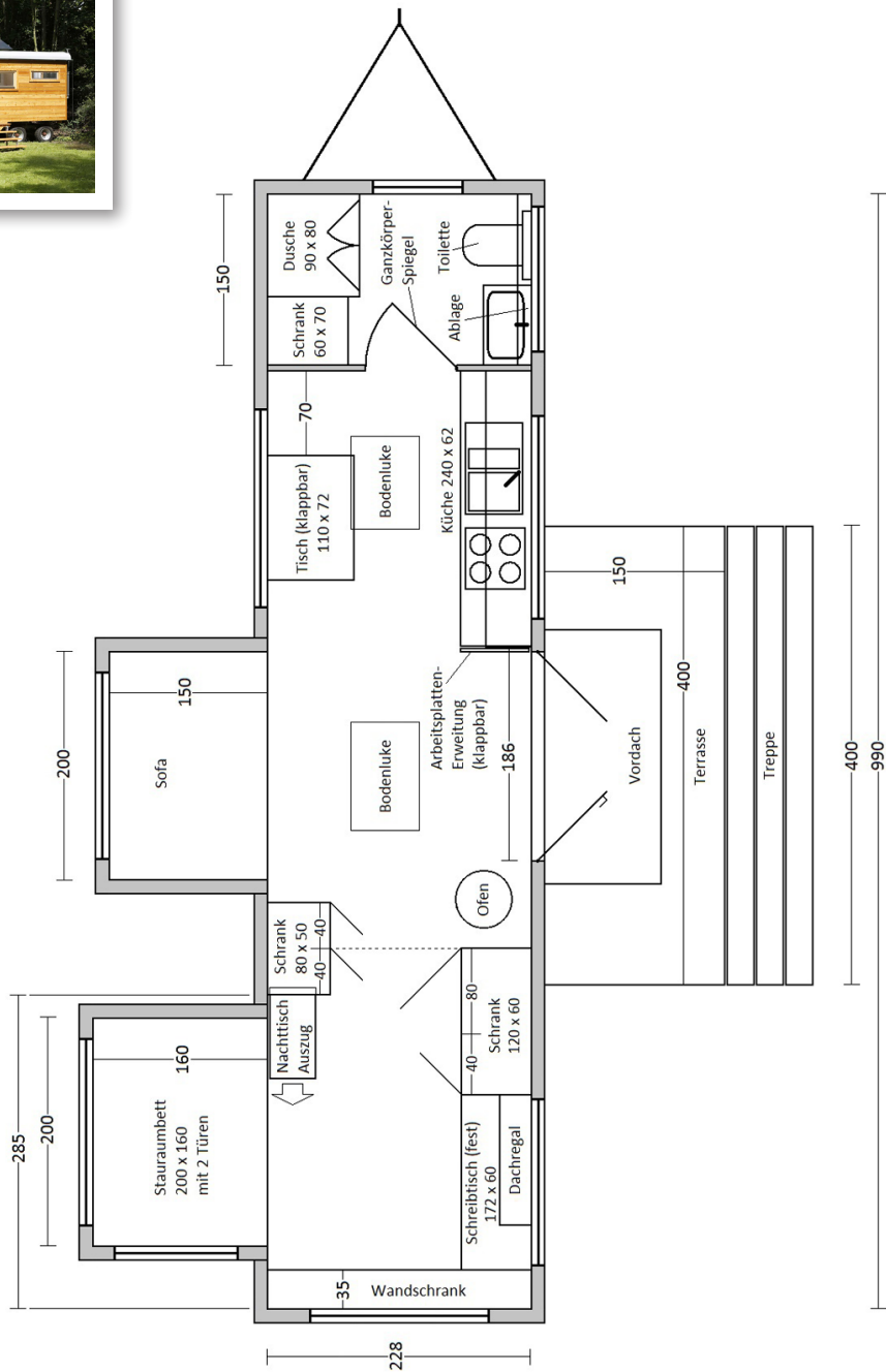
Grundriss Wohlwagen M2. Innenmaße in cm.
