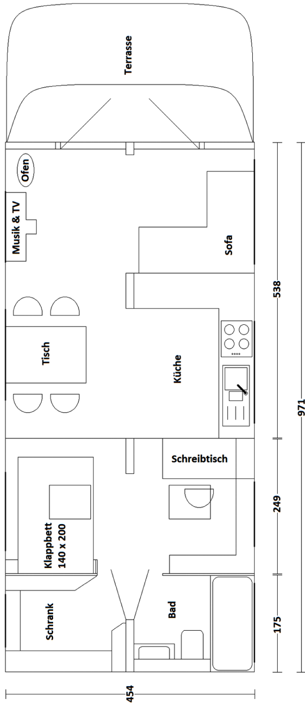
Grundriss Wohlwagen Multi. Innenmaße in cm.
